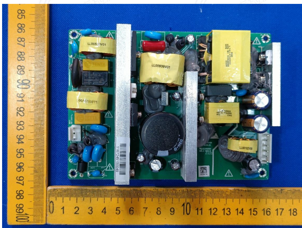
照片 10 内部电源正面
