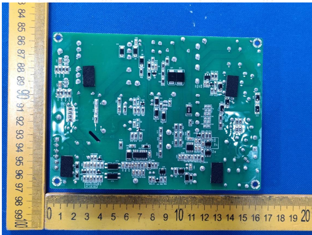
照片 11 内部电源反面
